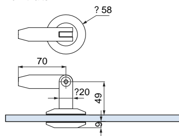
ES-G2083 E2 Fissaggio a punto sul vetro ? 58 Point fitting Punkthalter
