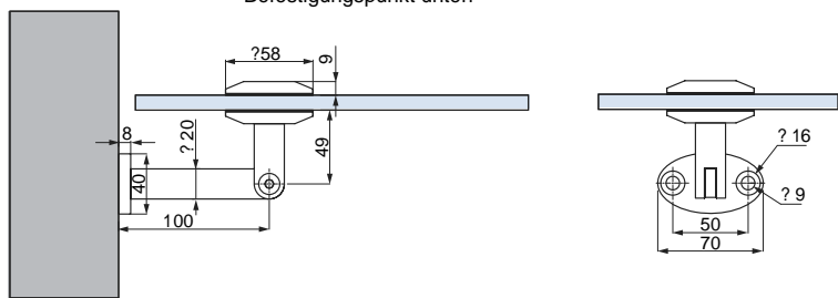
ES-G2083 E1 Punto di fissaggio inferiore Lower fastening point Befestigungspunkt unten
