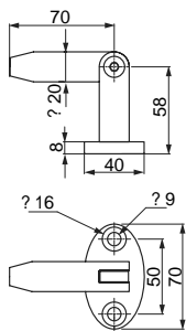
ES-G2083 E3 Punto di fissaggio superiore Upper fastening point Befestigungspunkt oben
